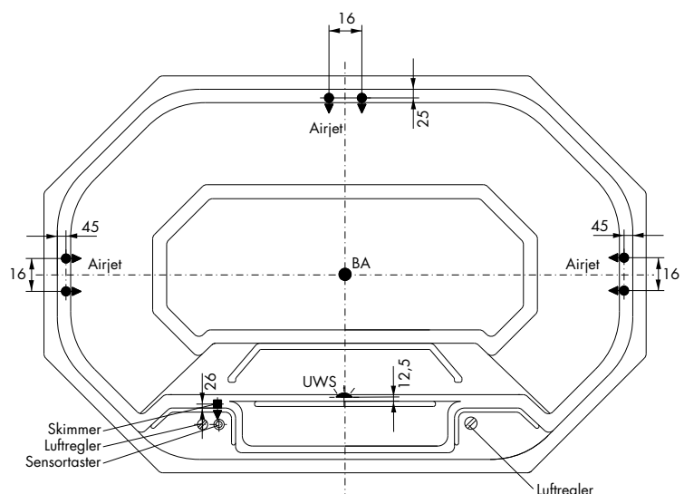
Standard-Positionen für Einbauteile
